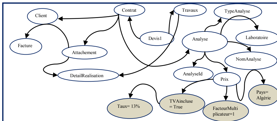
Figure.5. Extrait de l'ontologie locale de données (OLD) de la SETA (les concepts à l'intérieur des zones grisées représentent les informations contextuelles du concept 'Prix').
