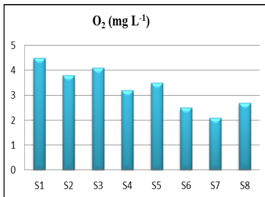
Figure. 5 : Variation des valeurs de l'Oxygène dissous
