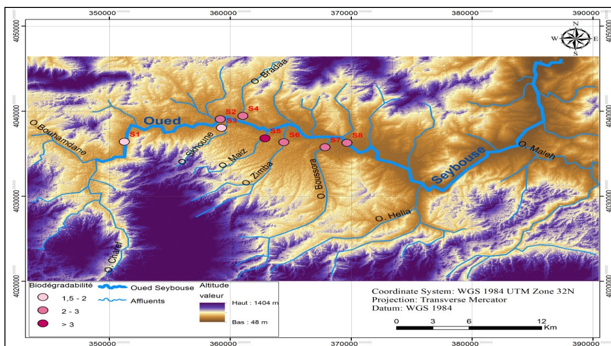
Figure. 12: Carte de la Biodégradabilité de la zone d'étude
