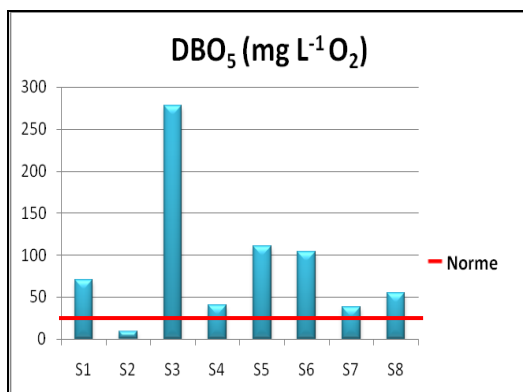
Figure. 6 : Variation des concentrations en DBO₅
