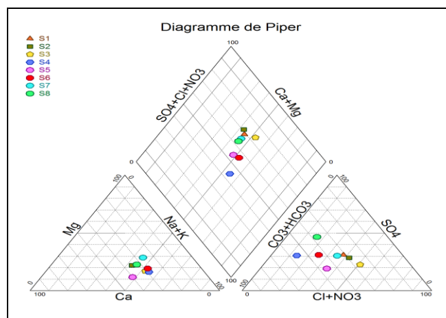
Figure 3 : Représentation graphique (diagramme de Piper)
