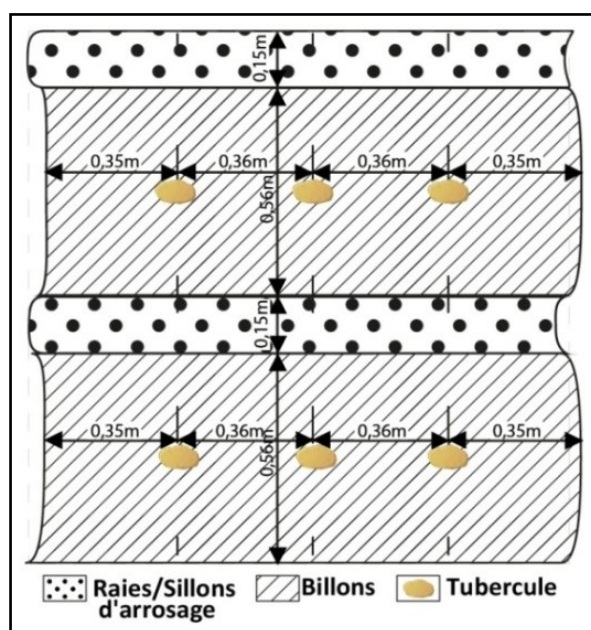
Figure 5 : Schéma de principe d'un carré d'essai
